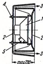
Rys. 10. Konstrukcja i wymiary głośnika typu GDT 51-54/10
