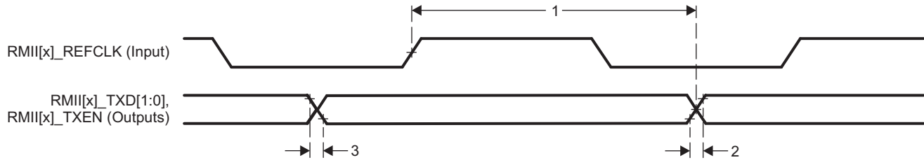
Figure 5-11. RMII[x]_TXD[1:0], RMII[x]_TXEN Timing - RMII Mode
