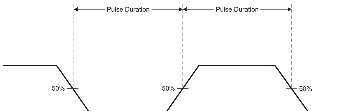
Figure 5-95. UART IrDA Pulse Parameters
