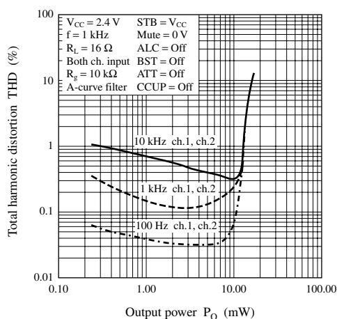
THD — P_O
