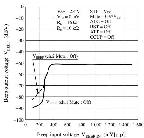
Beep — V_{IN}
