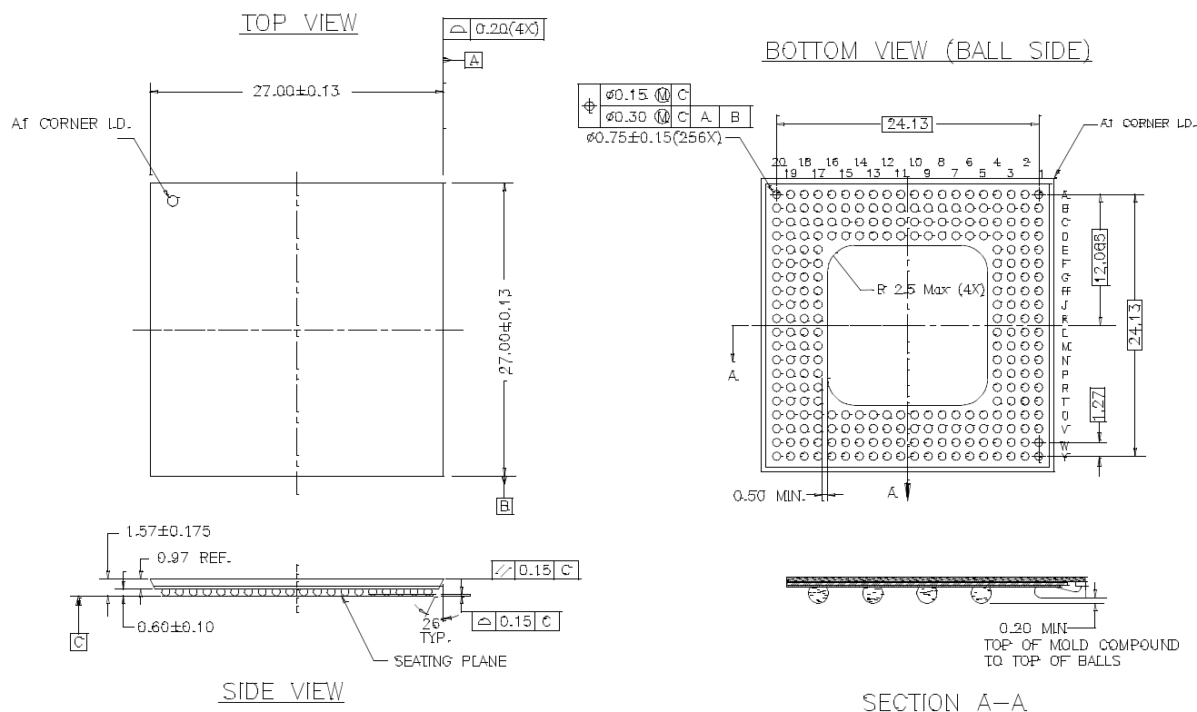
256-ball L2 Ball Grid Array (27 x 27 x 1.57 mm) BL256
