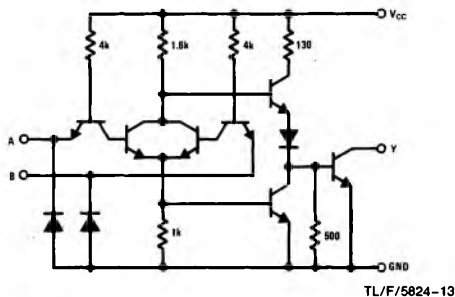
DS55453/DS75453
