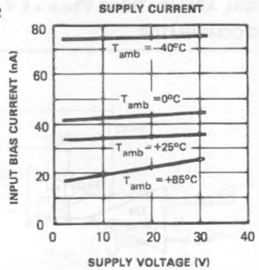
LM239,A LM2901-MC3302
