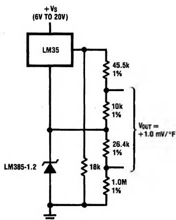
TL/H/5516-10 FIGURE 10. Fahrenheit Thermometer
