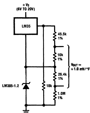
FIGURE 10. Fahrenheit Thermometer
