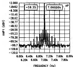
IMD 60 Hz, 7 kHz, 4:1
