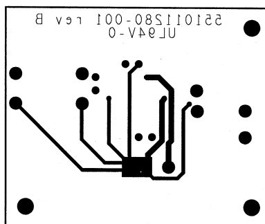
Figure 23. Bottom Layer
