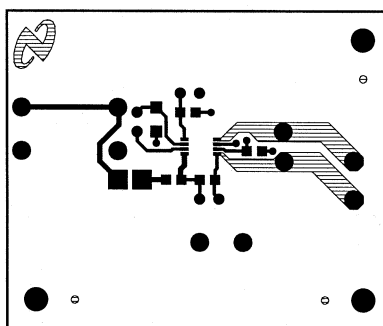
Figure 22. Top Layer
