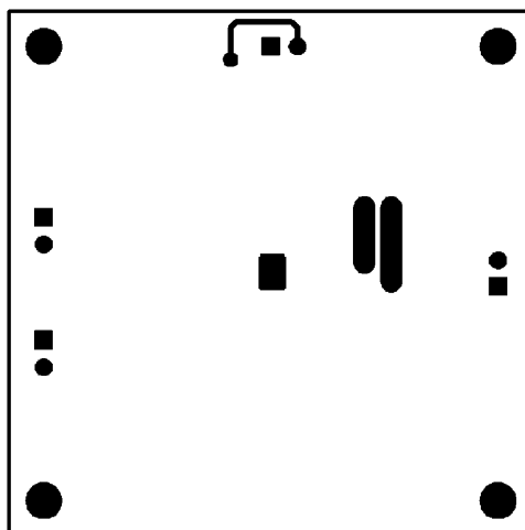
Figure 26. Bottom Layer
