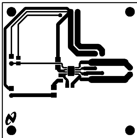
Figure 25. Top Layer
