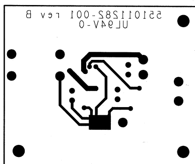
Figure 18. Bottom Layer
