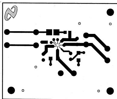
Figure 17. Top Layer
