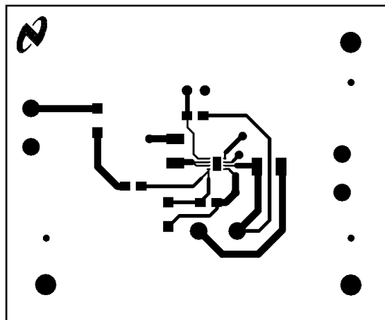
Figure 16. Top Layer
