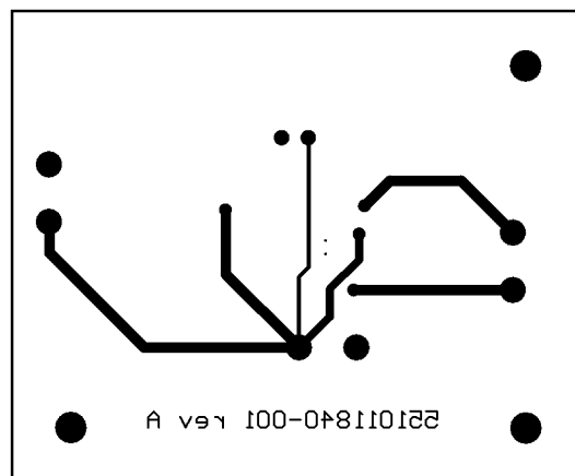
Figure 17. Bottom Layer
