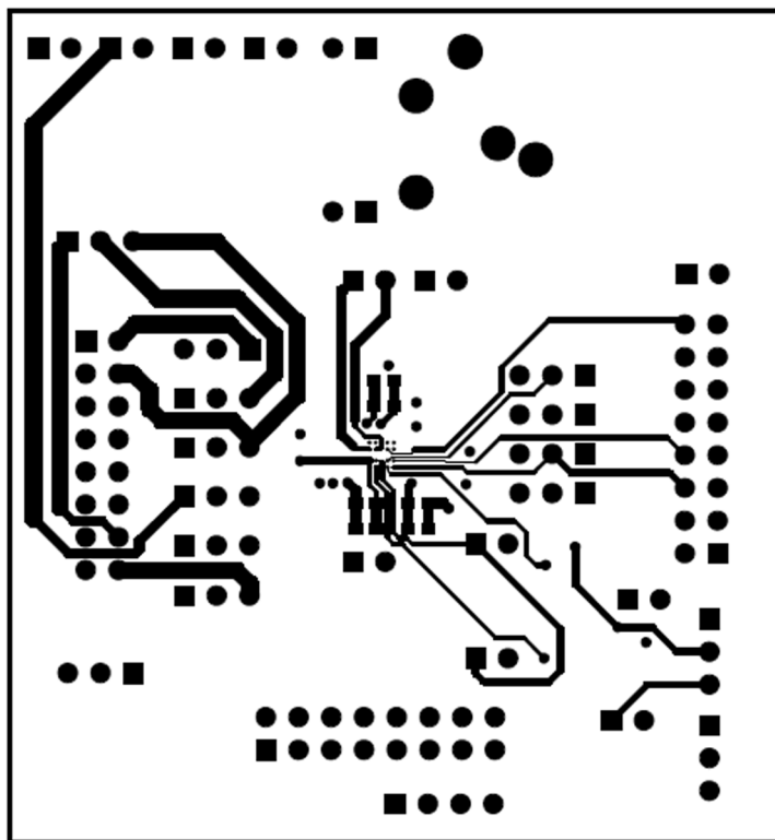
Figure 34. Bottom Layer
