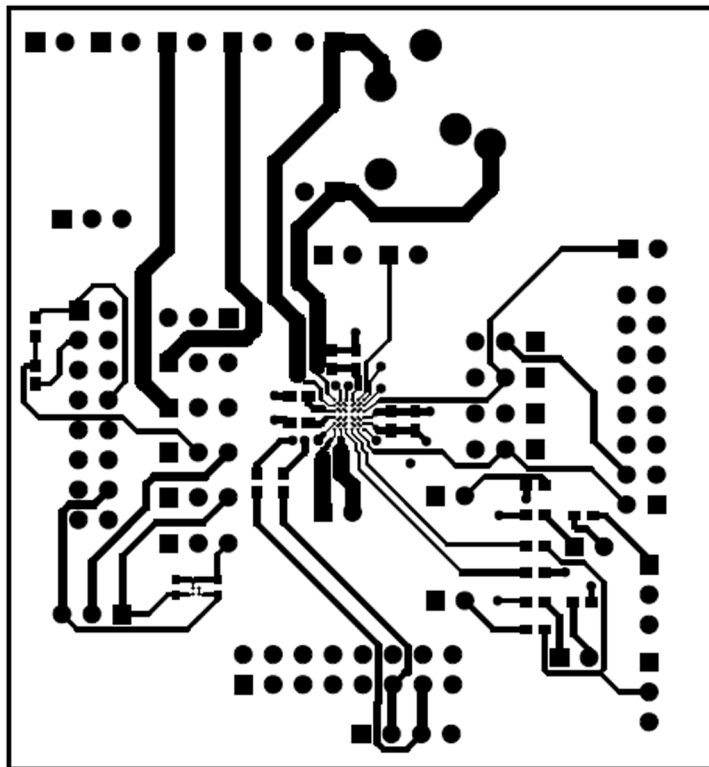
Figure 30. Top Layer
