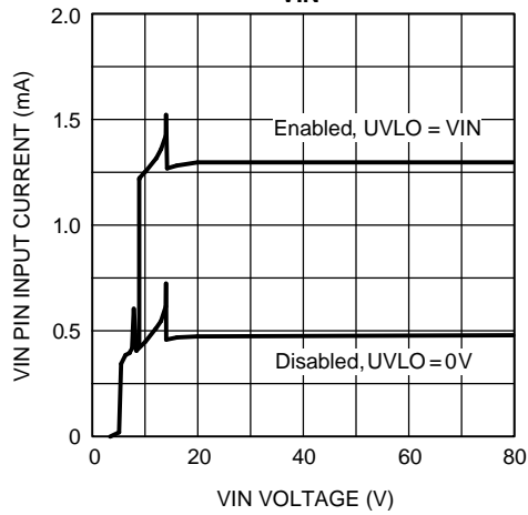
VIN Pin Input Current vs. VIN
