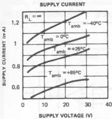
LM239,A LM2901-MC3302
