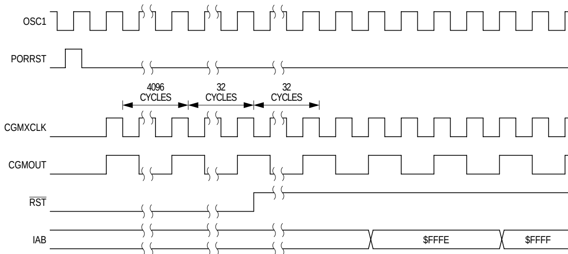
Figure 9-6. POR Recovery
