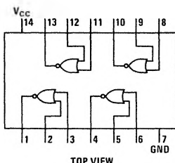
MM54C02/MM74C02
