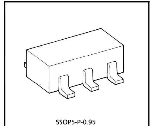
SSOP5-P-0.95 Weight : 0.014 g (Typ.)
