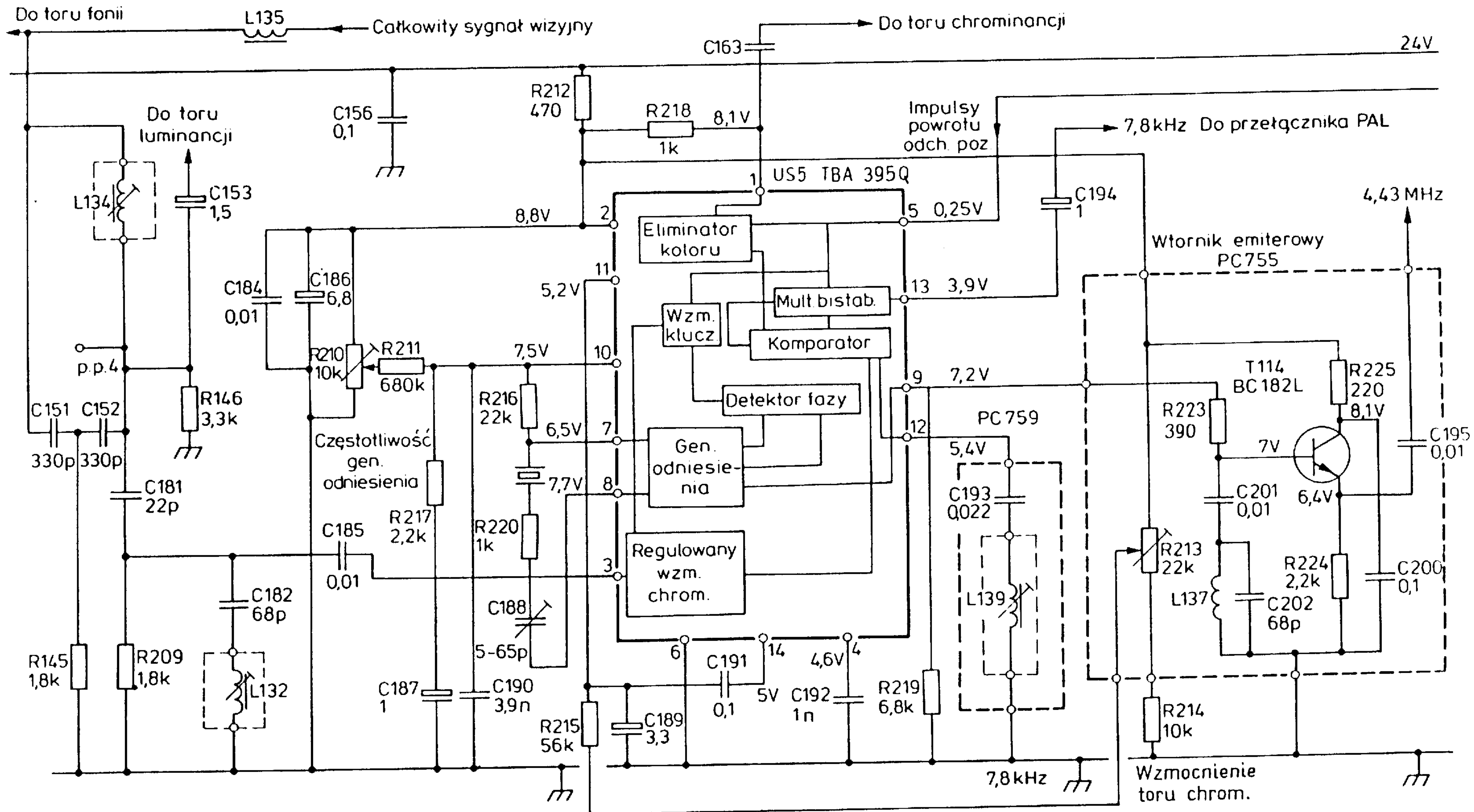
Rys. 11.5. Układ synchronizacji koloru z układem scalonym TBA 395Q (chassis 9000 firmy Ferguson)
