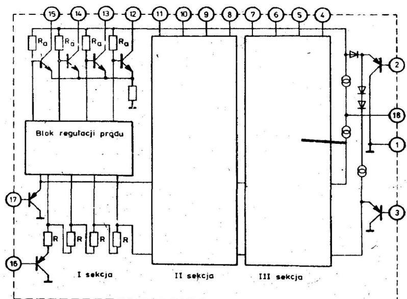
Schemat blokowy
