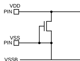
Fig. 4-9: Supply Pins (Power 1.8 V and Ground): VDDAC1 , VSSAC1 , VDDAC2 , VSSAC2 , VDDARGB , VSSARGB , VDDAFBL , VSSAFBL , VDDAPLL , VDDD1 , VSSS1 , VDDD2 , VSSS2 , VDDD3 , VSSS3 , VDDD4 , VSSS4
