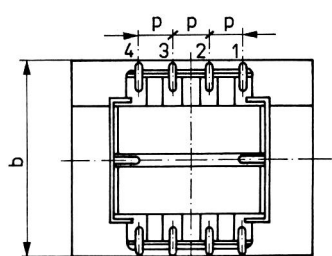
Położenie końcówek poz. 2 i 3
