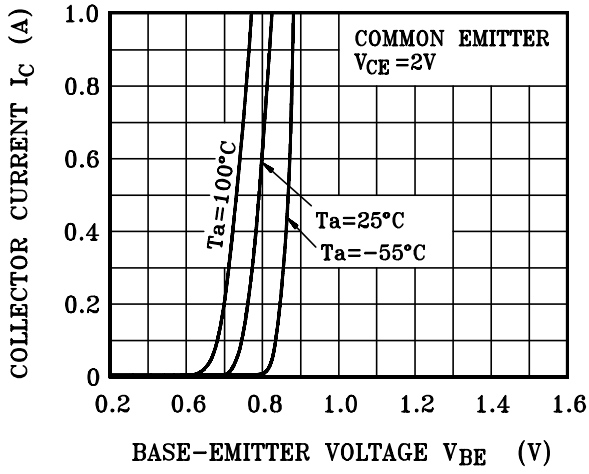
I_C - V_{BE}
