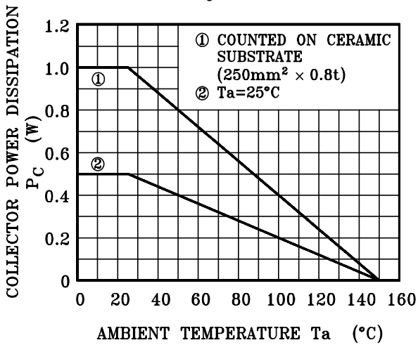
P_C - T_a
