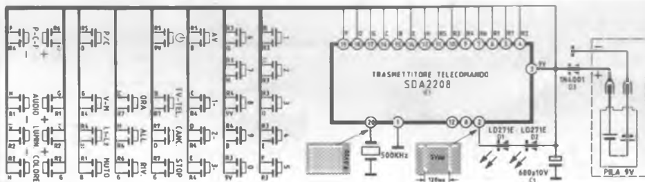
TV3629 - TRASMETTITORE INFRAROSSI TC3
