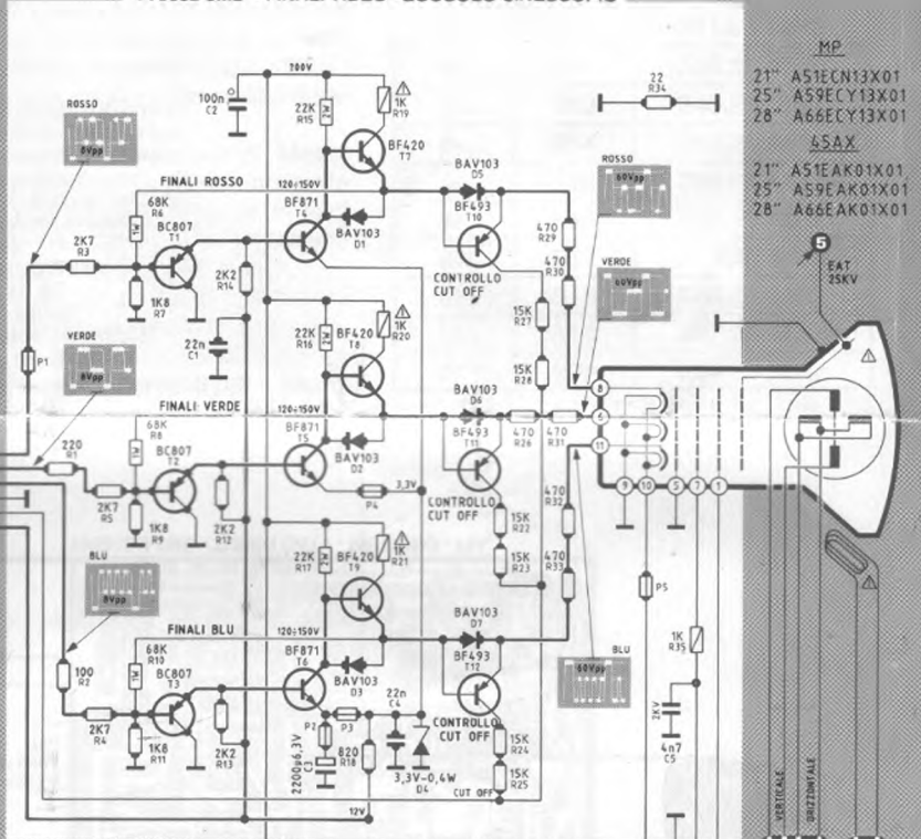
CONNETTORE n°10 Aim Finali Video
