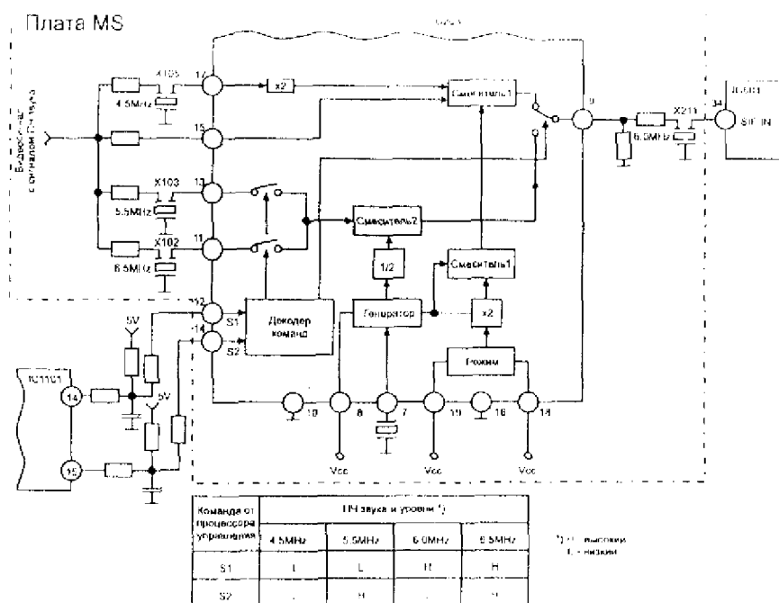
Рис. 2.15. Структурная схема прохождения сигналов ПЧ Звукa через плату MS
