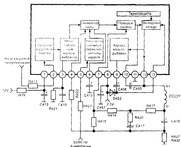
Рис. 2.24. Структурная схема микросхемы LA7837 и способ ее включения в шасси MX-3C
