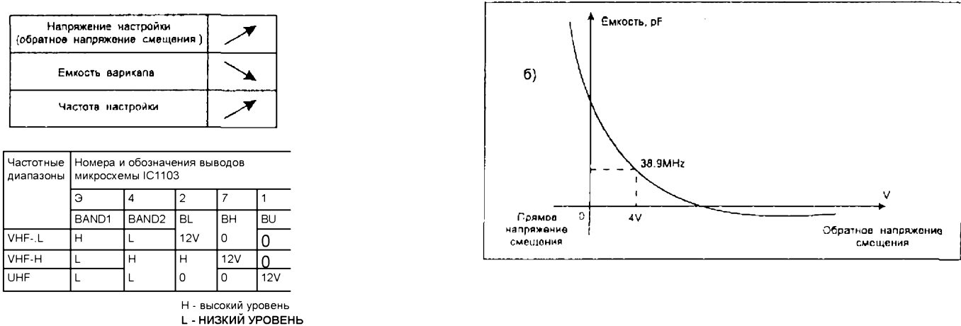
Рис. 2.11. К пояснению способов настройки (а, б) и переключения диапазонов (в) тюнера
