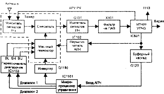
Рис. 2.10. Структурная схема радиоканала
