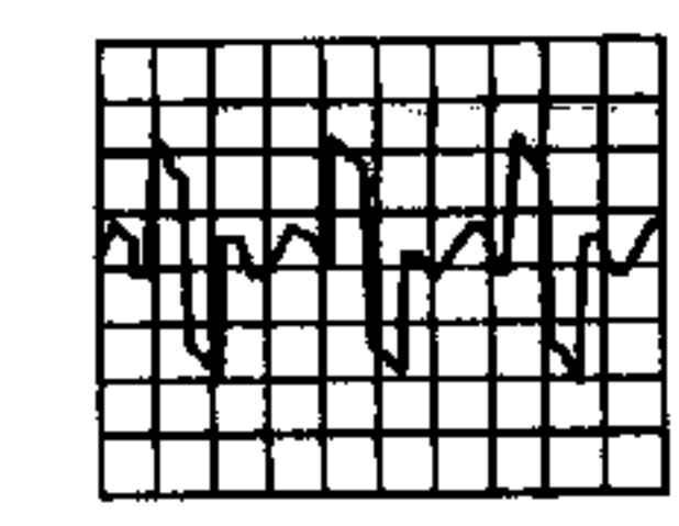
TP 29 ① 0,1V/div AC 20 uS/div
