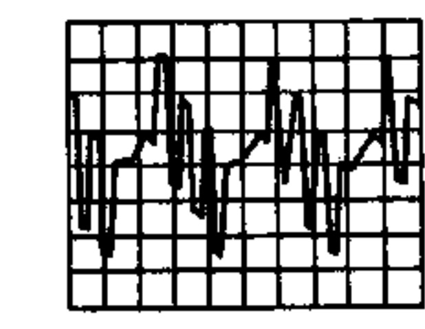
TP 30 ① 0,1 V/div AC 20 uS/div
