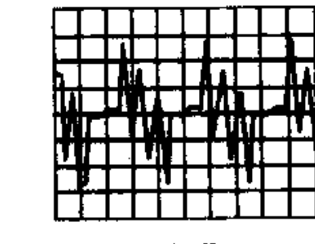
TP 31 ① 0,2 V/div AC 20 uS/DIV
