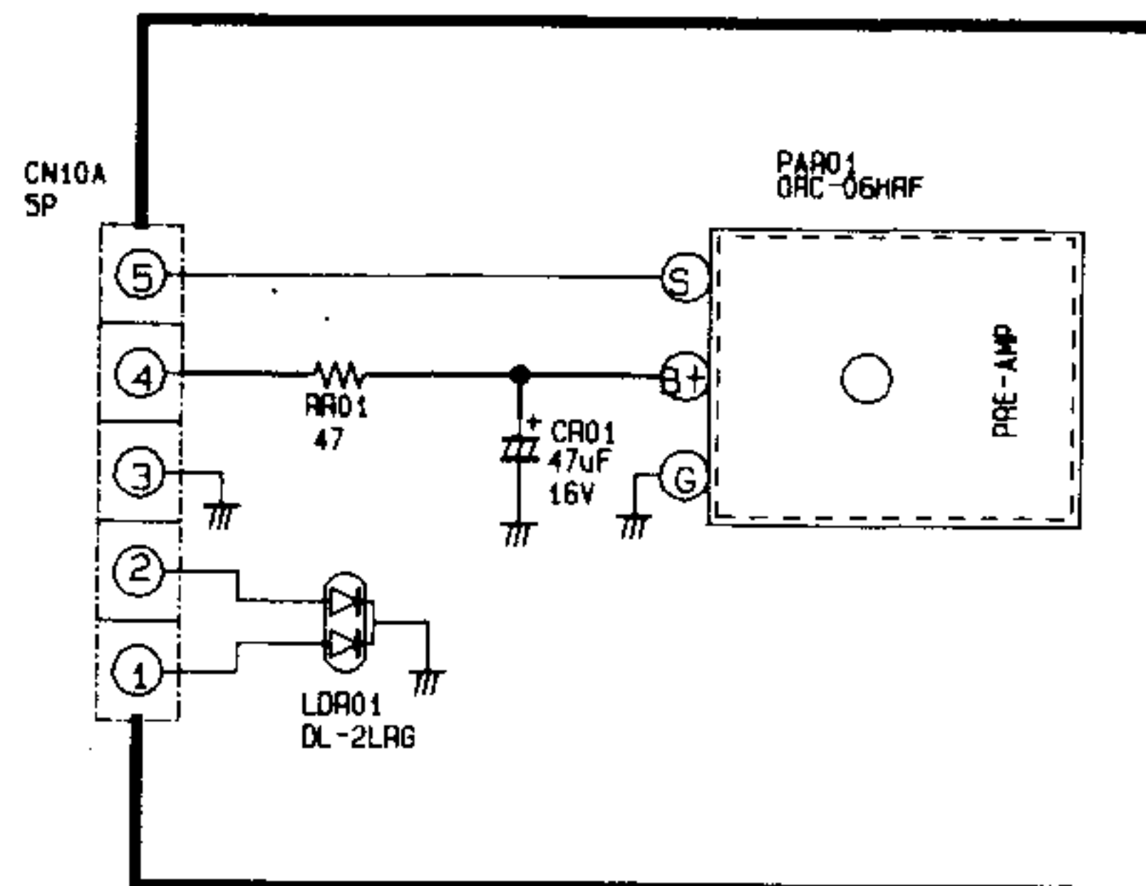
RICEVITORE TELECOMANDO
