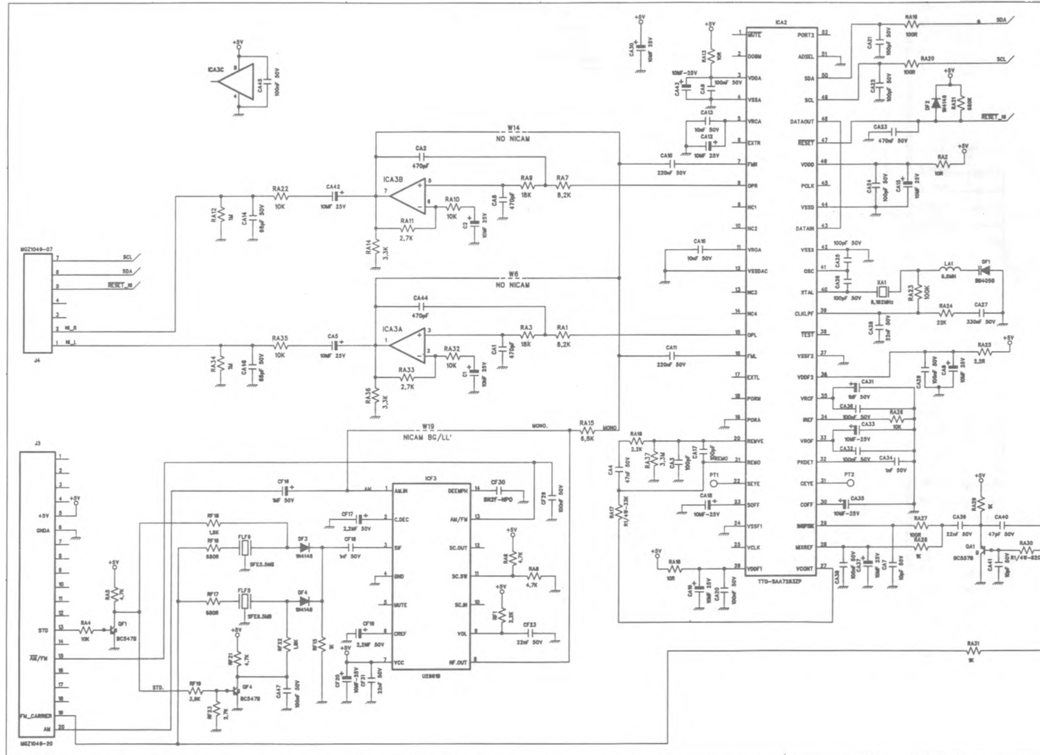
NICAM STEREO DEVRE ŞEMASI
