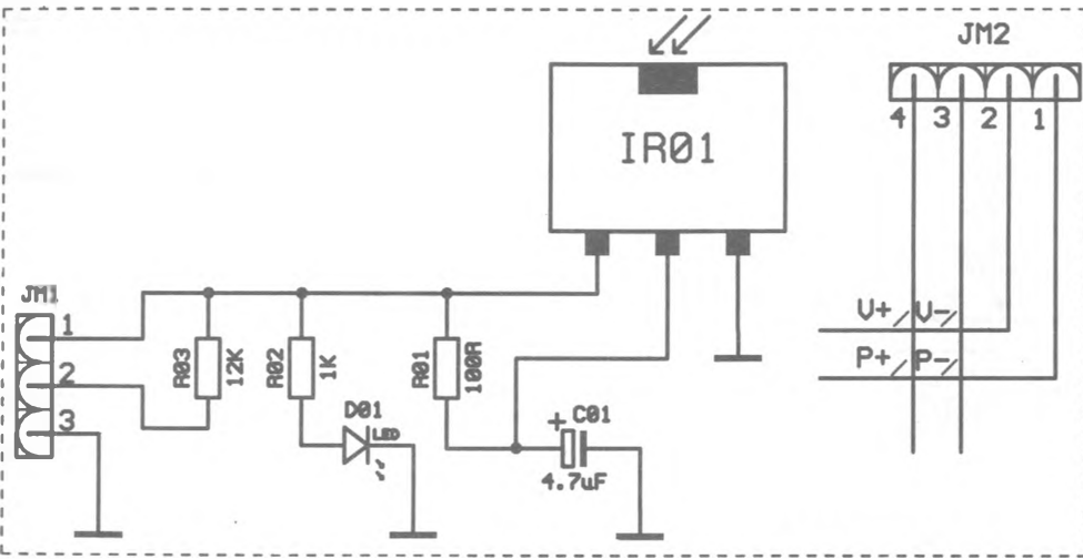
TUŞ TAKIMI DEVRE ŞEMASI
