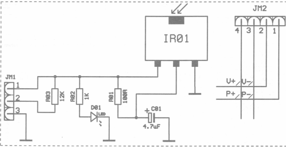
TUŞ TAKIMI DEVRE ŞEMASI
