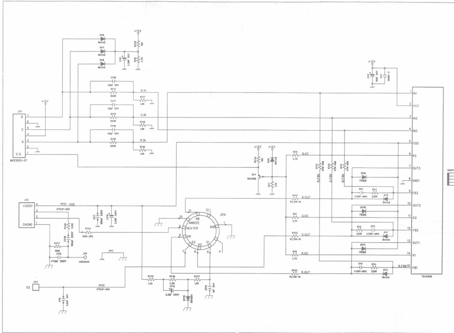
TÜP SOKETİ DEVRE ŞEMASI
